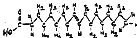
OLEIC ACID
