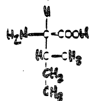
SELEUCINE
