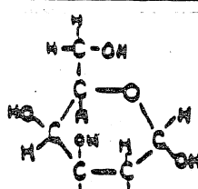
GALACTOSE
