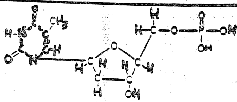
DEOXYRIBOSE THYMINE
