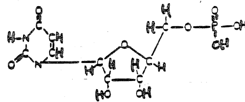
RIBOSE URACIL
