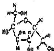
FRUCTOSE
