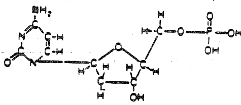
DEOXYRIBOSE CYTOSINE
